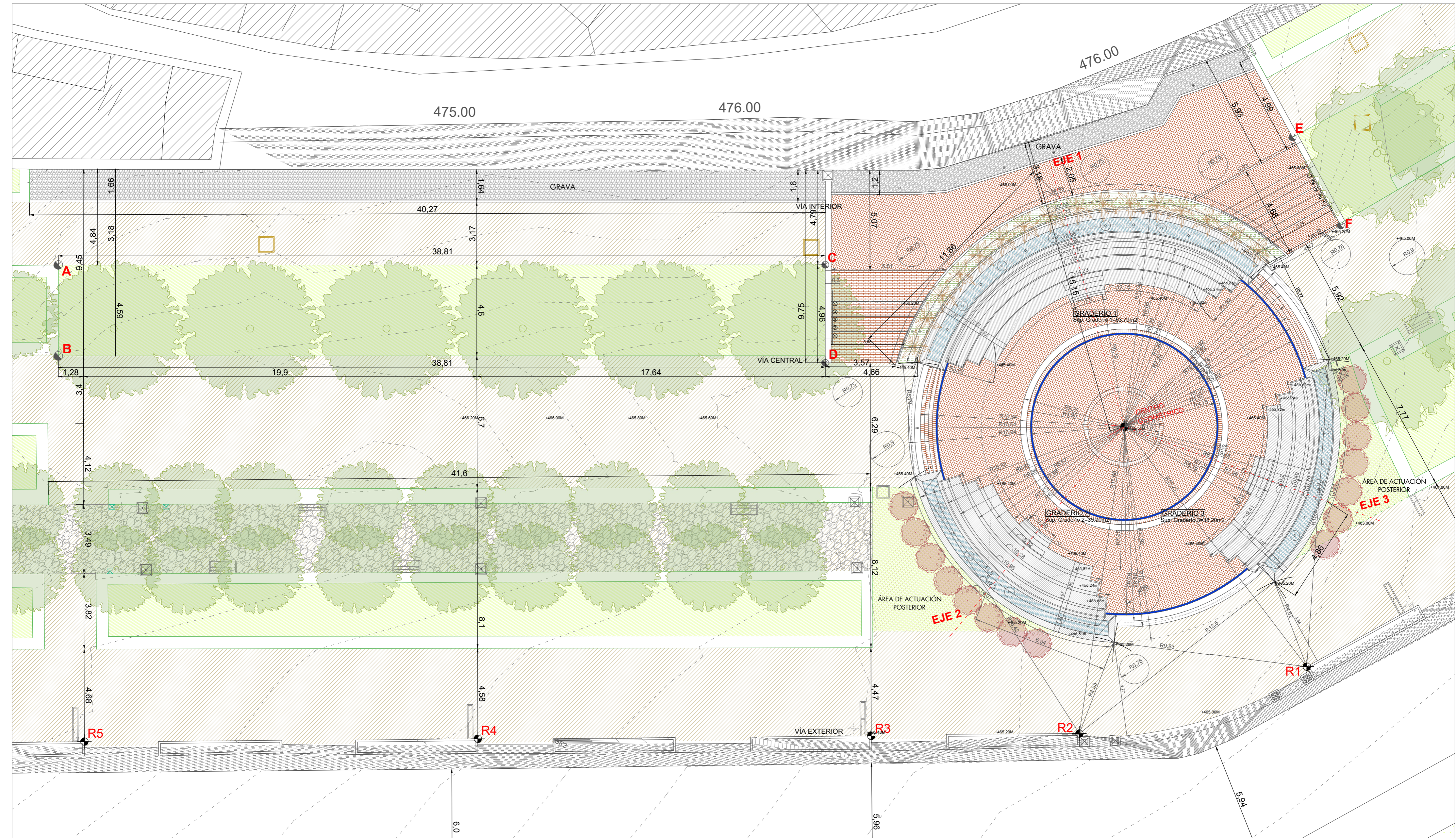
PLANTA PARQUE DE SANTA LUCÍA | ZONA DE ACTUACIÓN E 1:125
